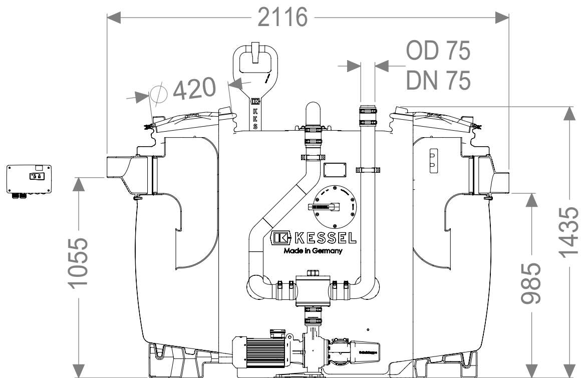
A-A (1 : 20)
