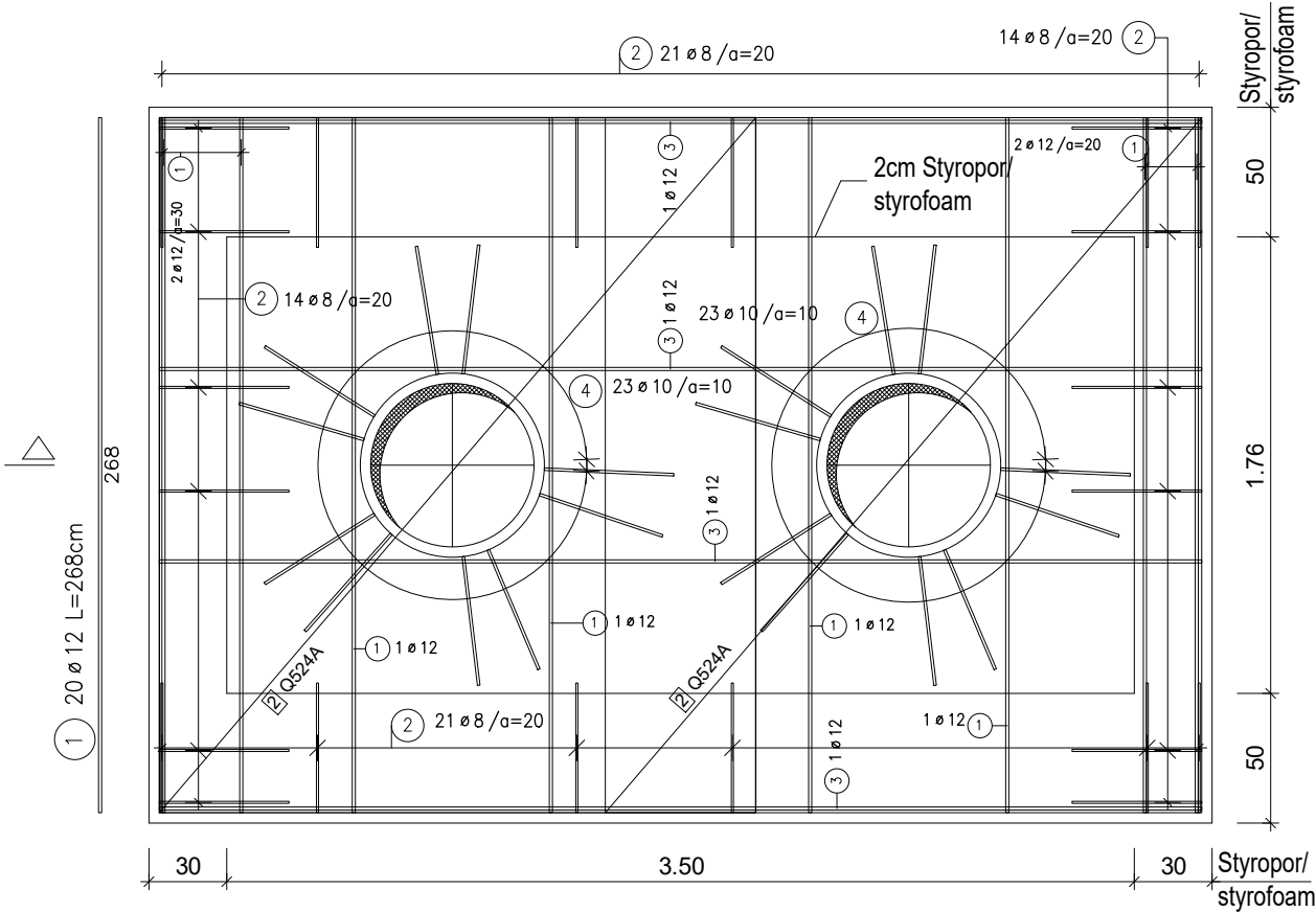
Untersicht
