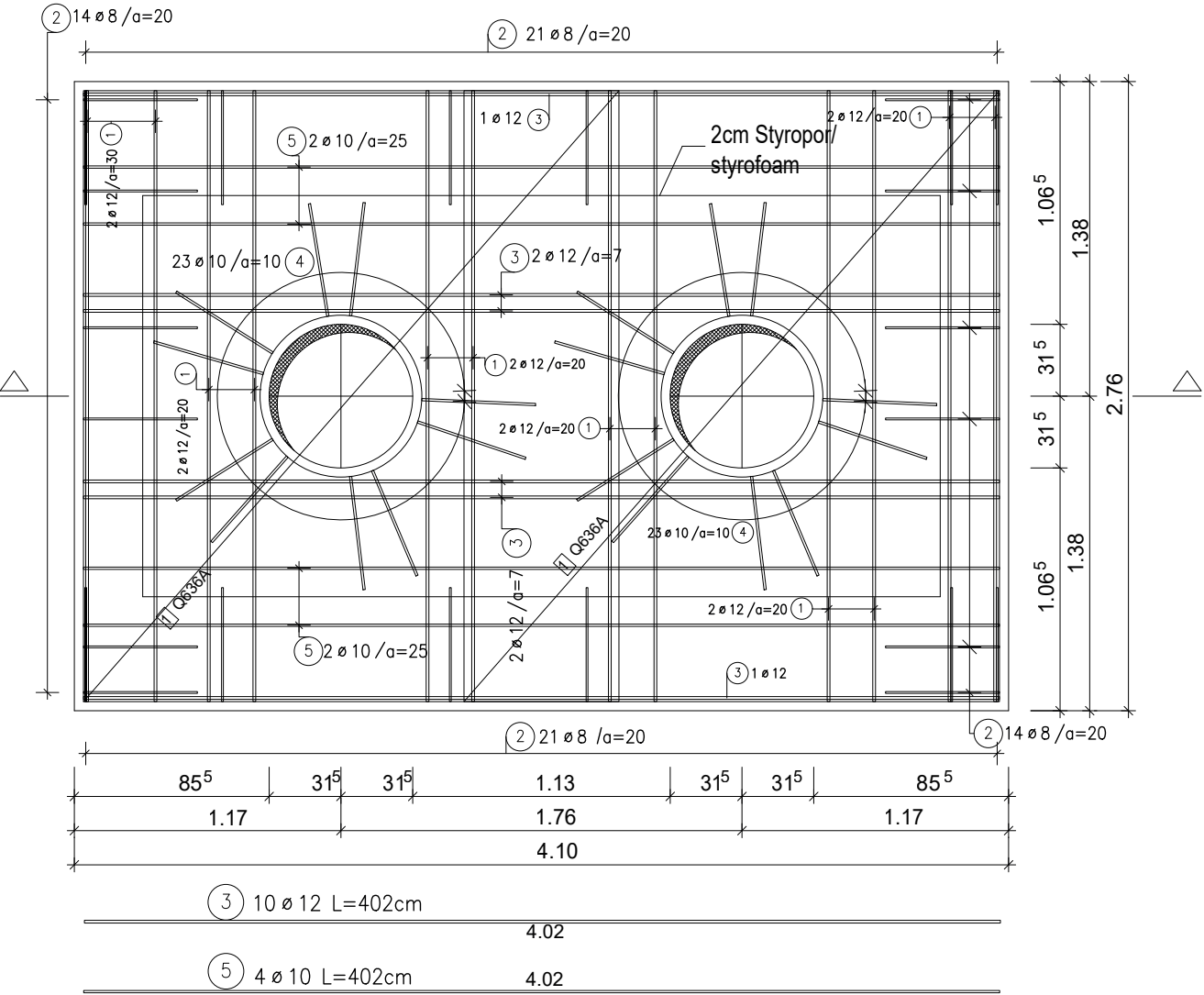
Draufsicht
