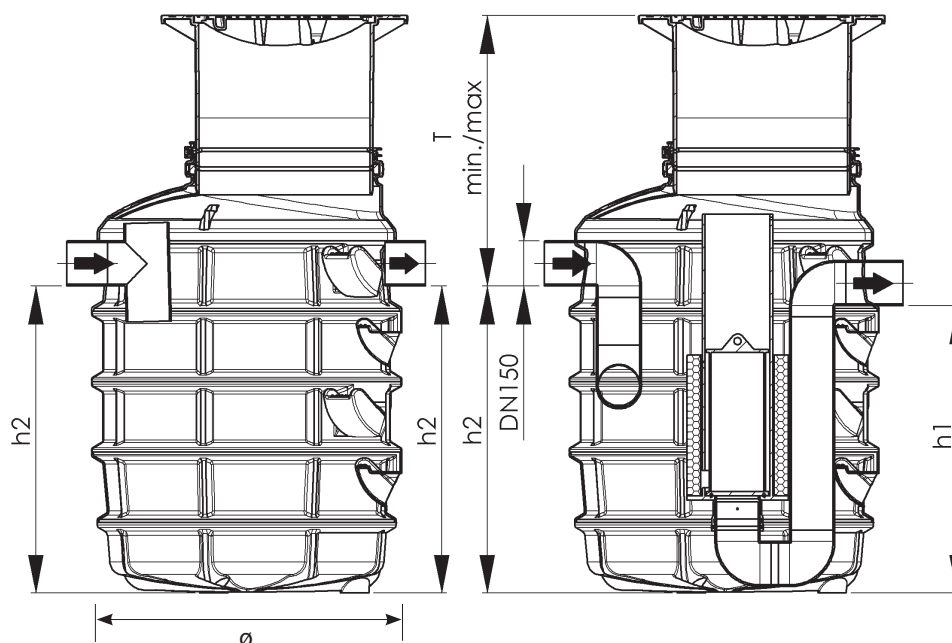
3.7 Måttitning KESSEL-koalescensavskiljare EasyOil FB 1000, NS 6 (med separat slamfång)
