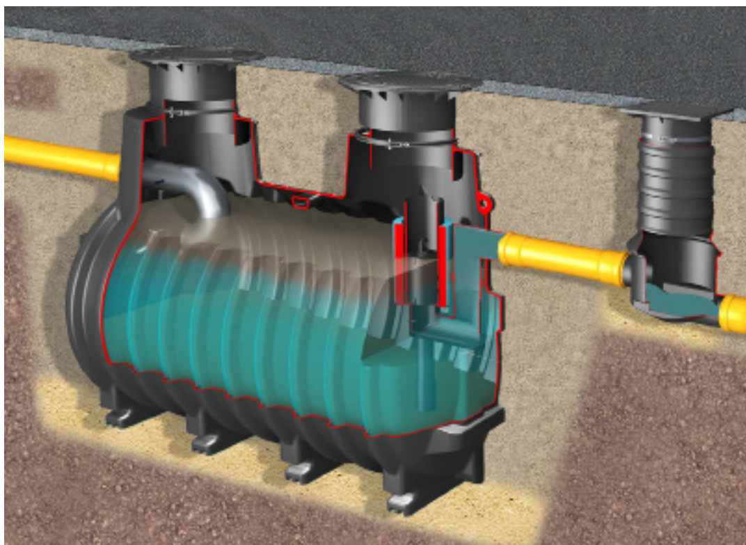
Bilden visar KESSEL-koalescensavskiljarcistern EasyOil System A med betäckning klass B och provtagningsbrunn
