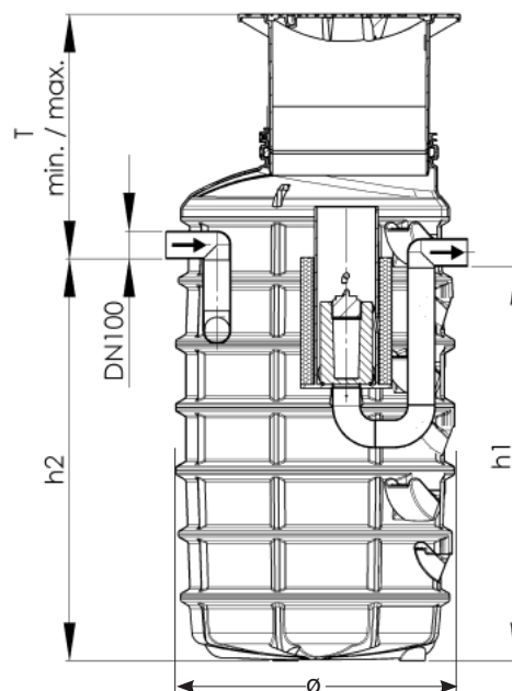
3.6 Måttitning KESSEL-koalescensavskiljare EasyOil schakt FB 1000, NS 3
