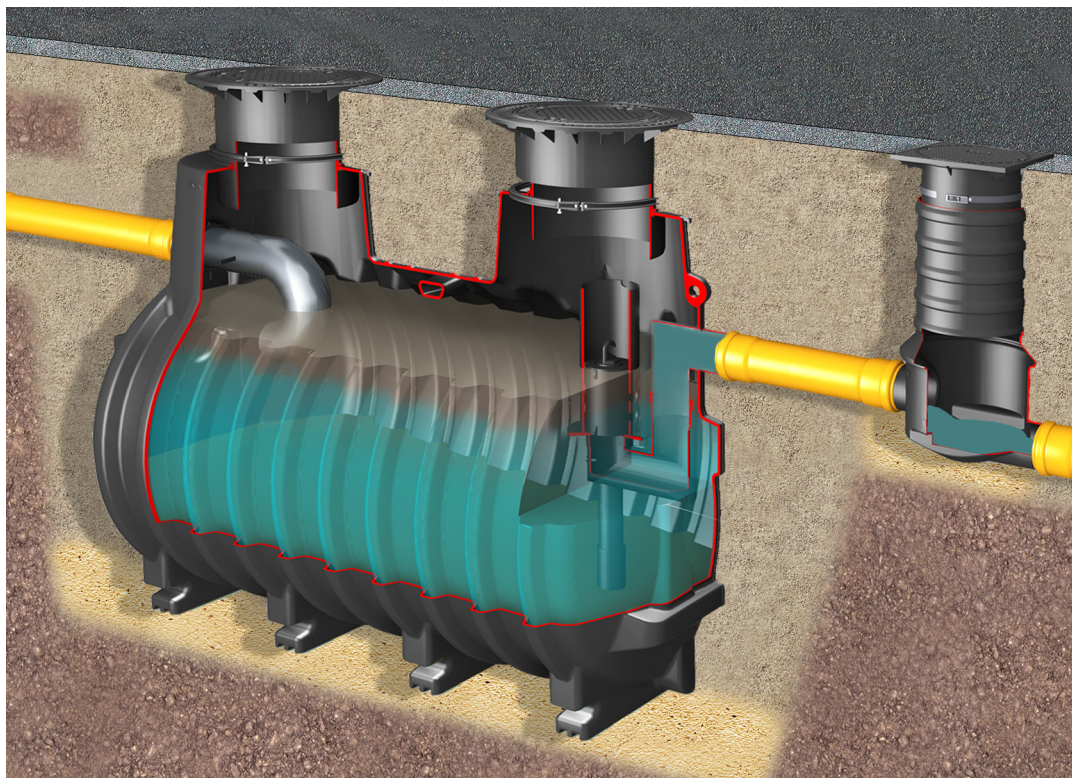
Bilden visar KESSEL-olje-/bensinavskiljarcistern EasyOil med betäckning system B och provtagningsbrunn
