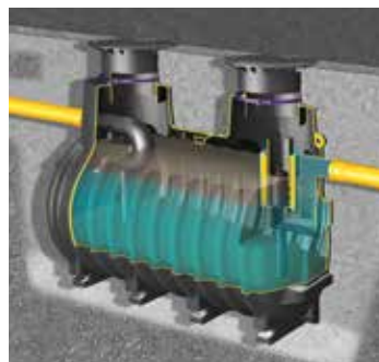
Koaleszenzabscheider EasyOil
