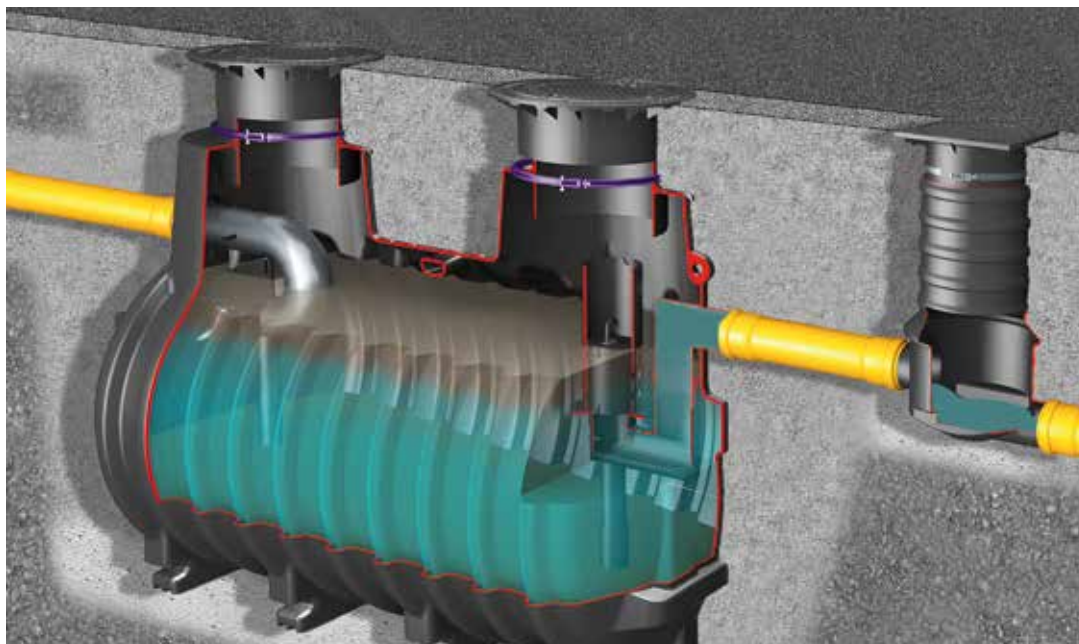
Koaleszenzabscheider mit Probenahmeschacht
